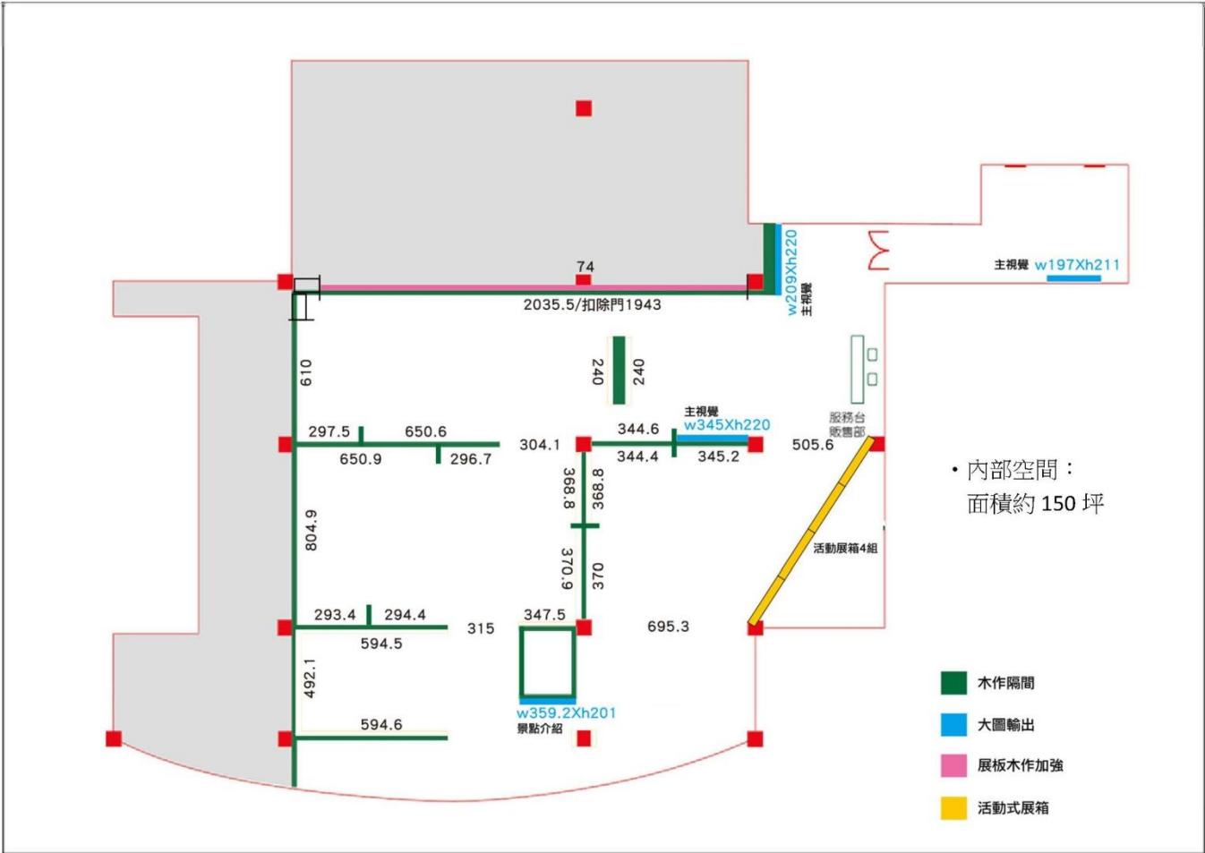
滬水一方藝文空間(5 樓平面圖)
