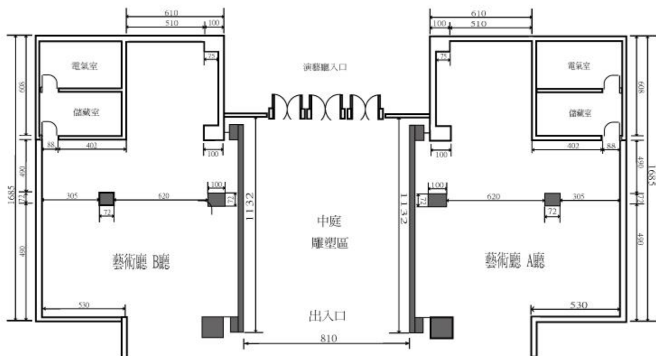
新莊文化藝術中心展覽場地平面圖
