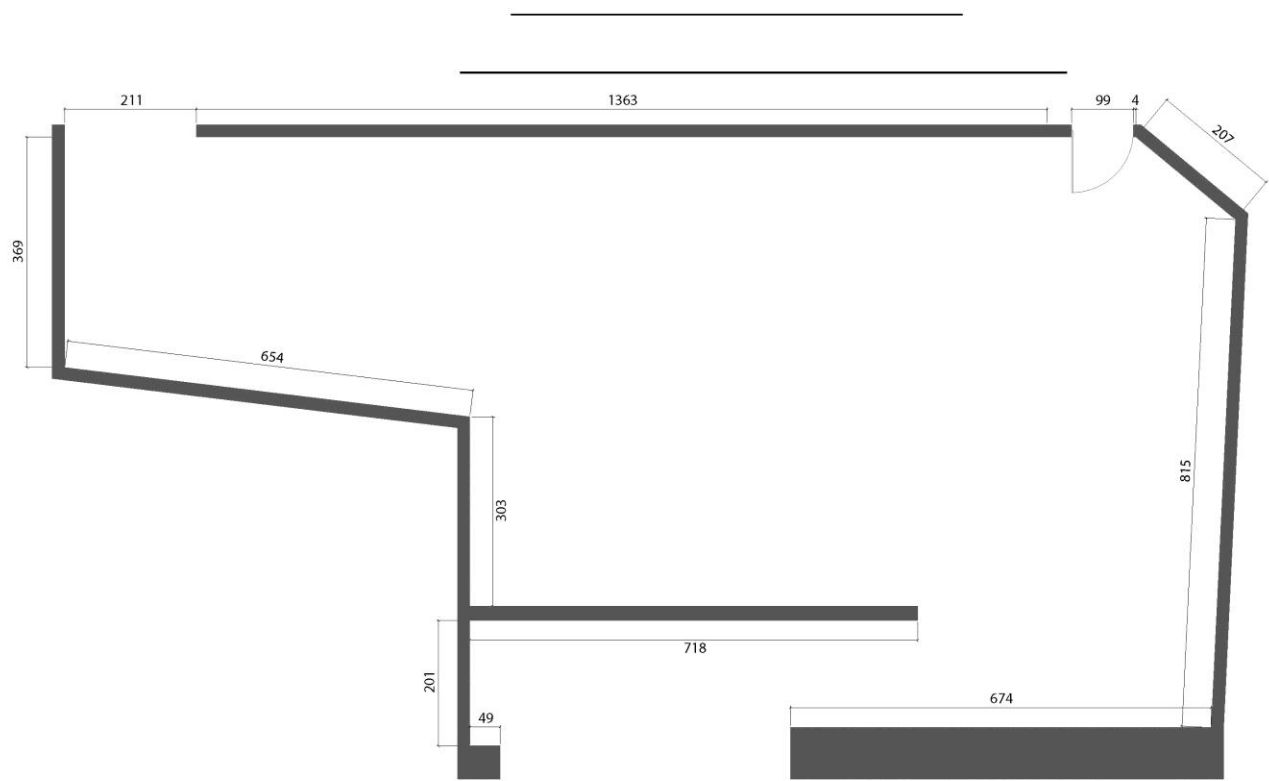
4F平面配置圖
