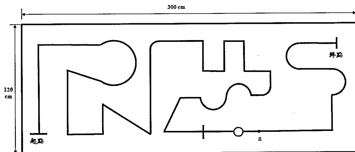
自走車循跡避障比賽場參考地圖
