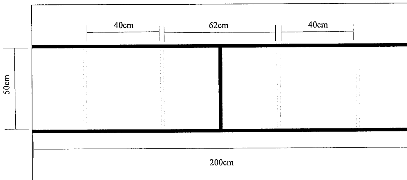
【圖一】拔河機器人競賽場地
