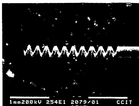
圖二 微細彈簧螺 SEM 圖
