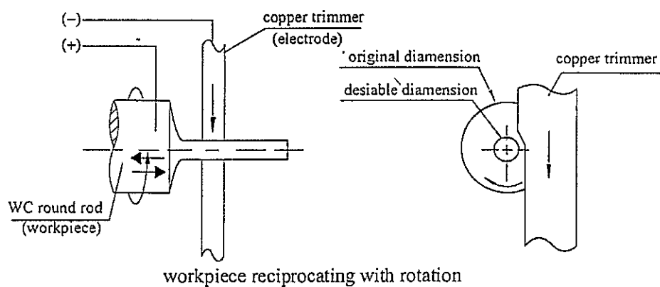
圖一 微細圓形電極之加工示意圖
